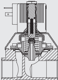
Schnittzeichnung
